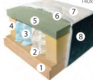
POPREČNI PRESEK KORLEONE DELUX
