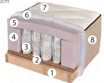
POPREČNI PRESEK KORLEONE
